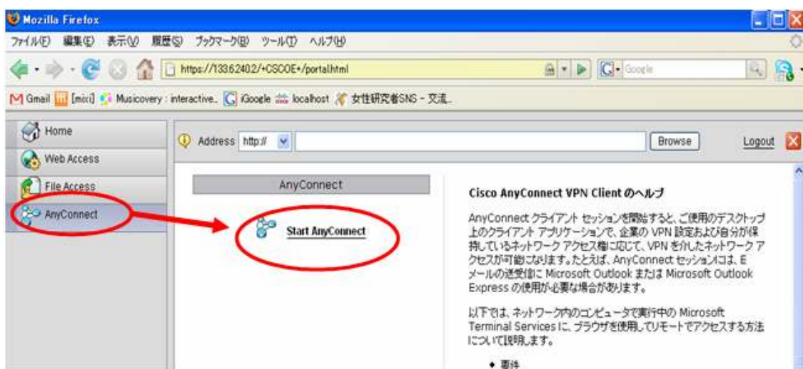
図1：AnyConnect の起動
